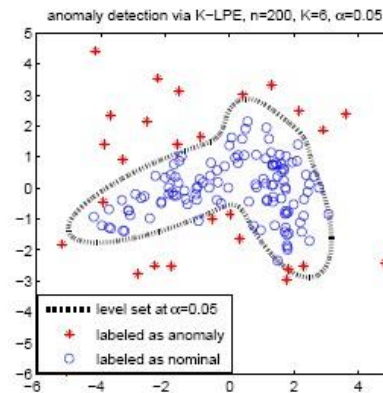
异常检测
