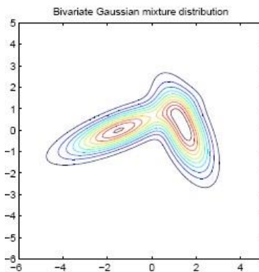
异常检测
