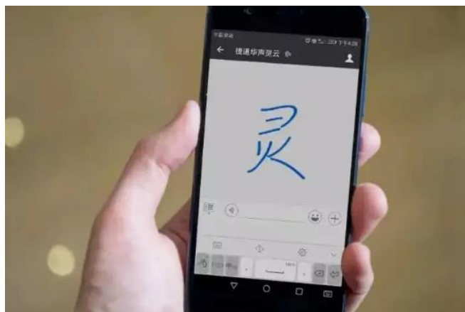
手写识别
