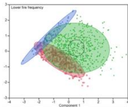
聚类
