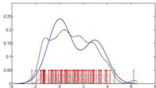
密度估计
